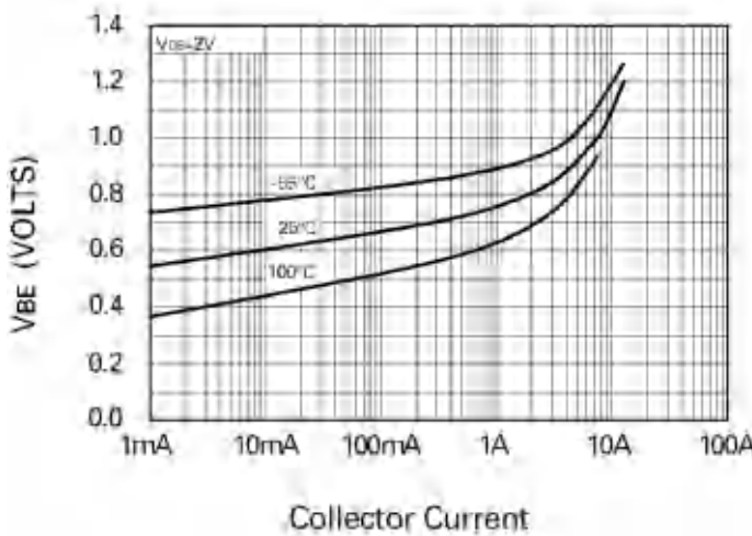
VBE(ON) vs IC
